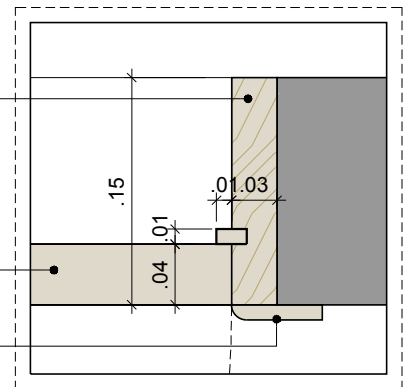
DET - 01 ESCALA 1/5
