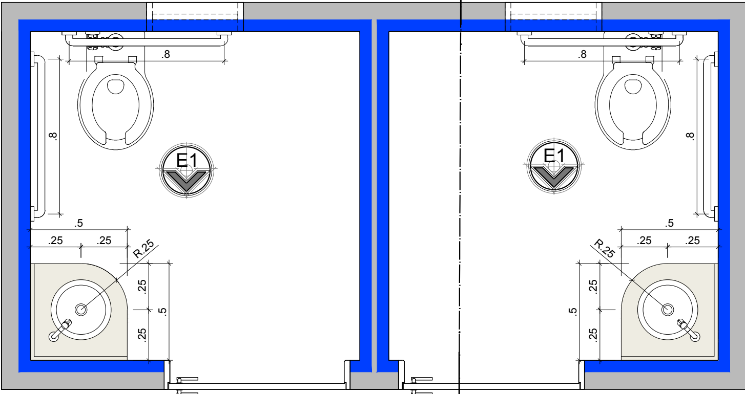
PLANTA BAIXA - WCS ESCALA 1/20
