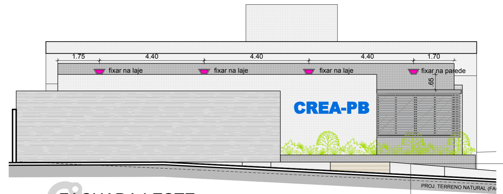
FACHADA LESTE ESCALA 1/100
