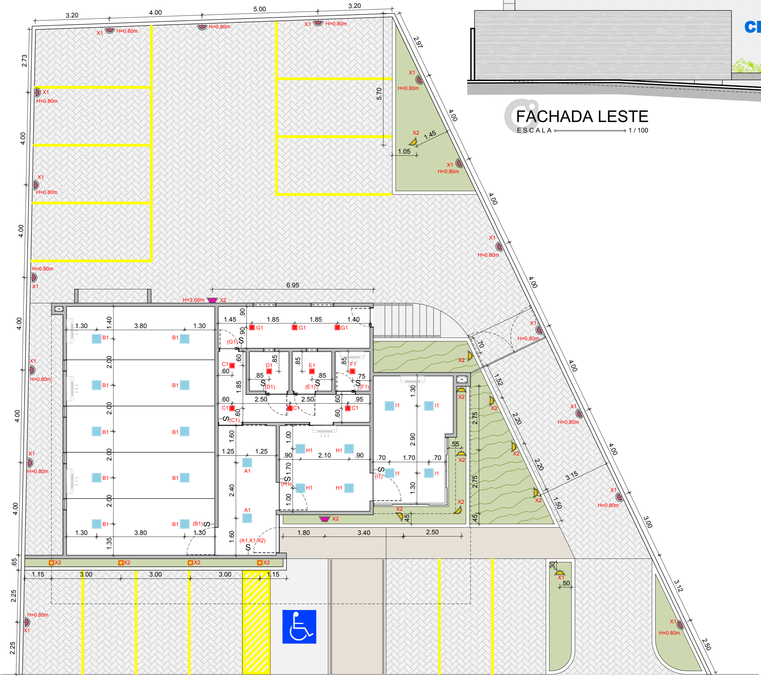
PLANTA BAIXA - LUMINOTÉCNICO ESCALA 1/100
