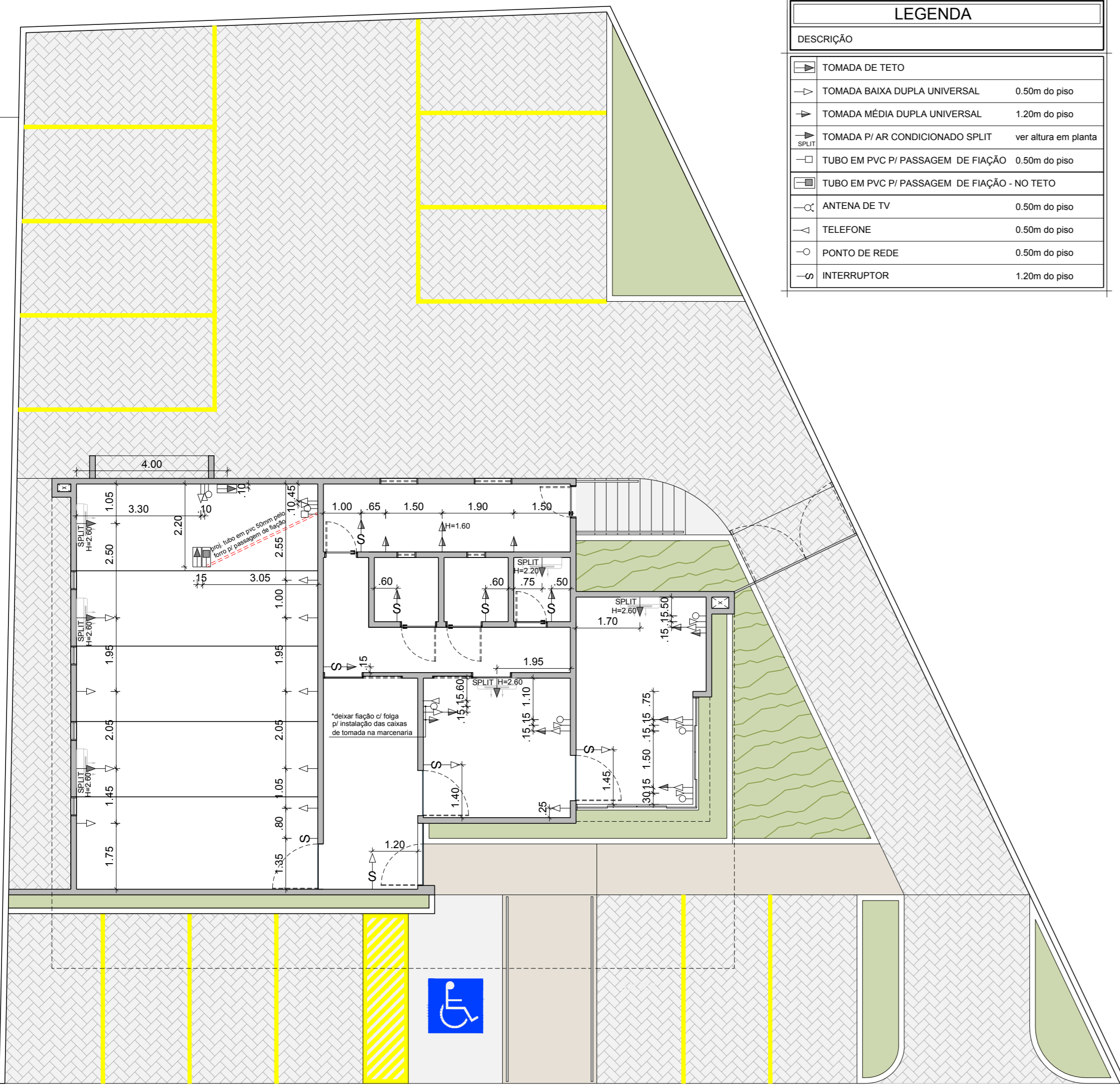
PLANTA BAIXA - ELÉTRICO ESCALA 1/100
