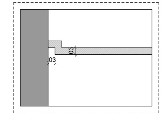
DETALHE - 01 ESCALA 1/10 CANTONEIRA
