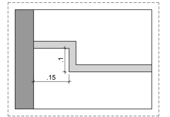
DETALHE - 02 ESCALA 1/10 CORTINEIRO
