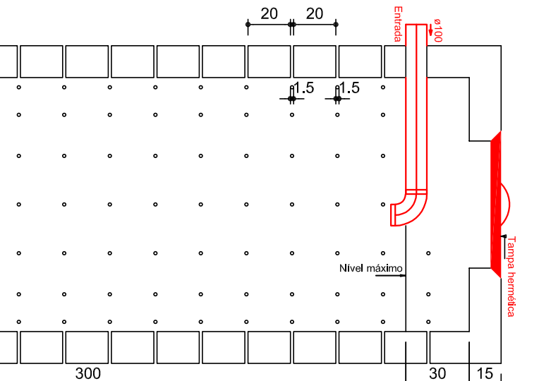
SUMIDOURO
