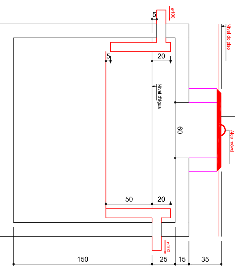
TANQUE SÉPTICO
