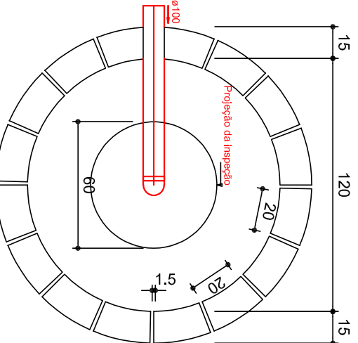
SUMIDOURO
